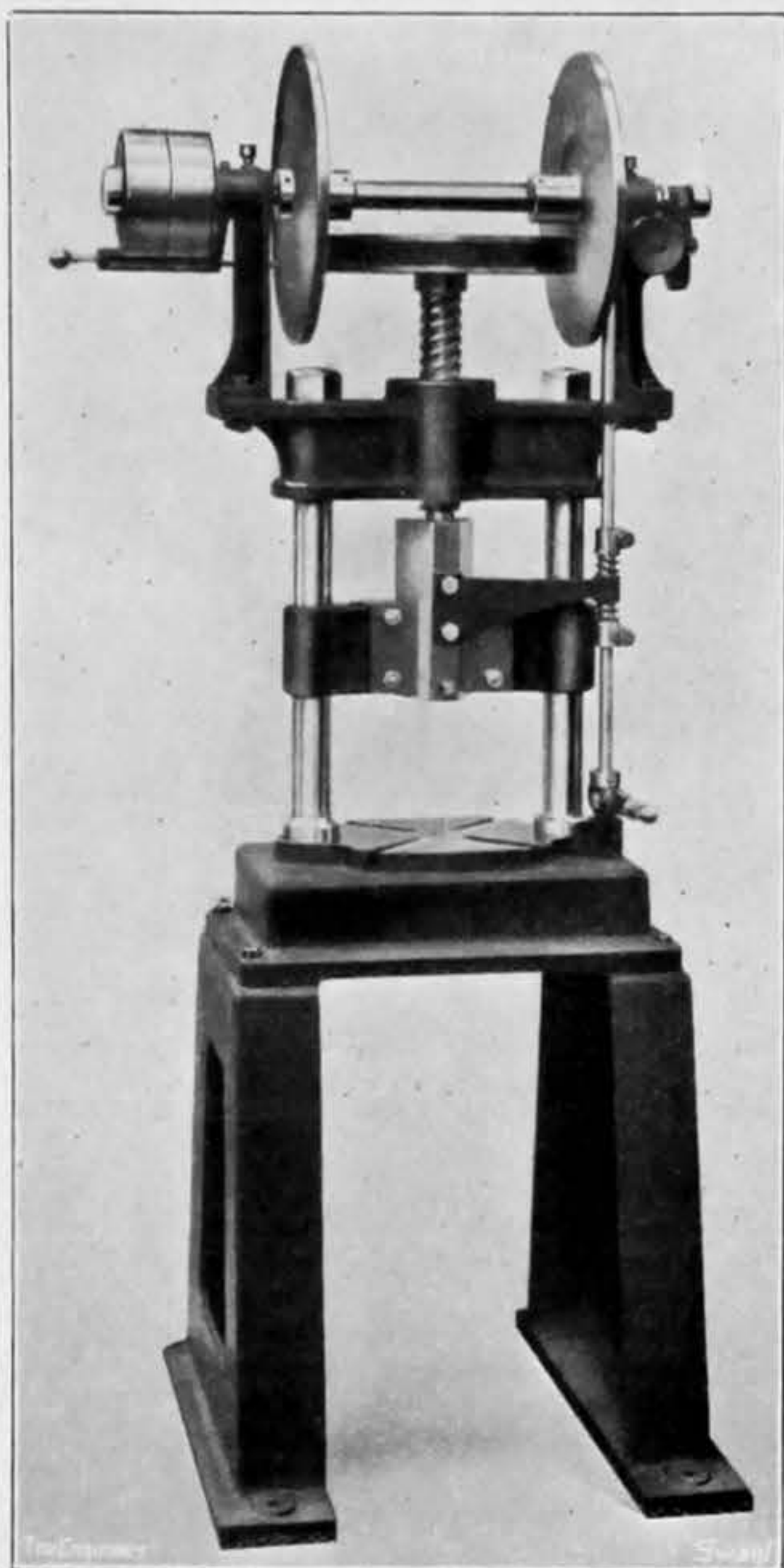
FIG. 14—FRICTION-DRIVEN SCREW PRESS
